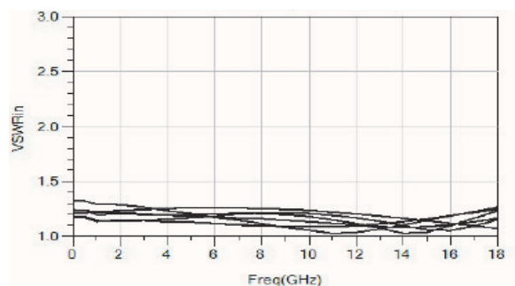
输入驻波
