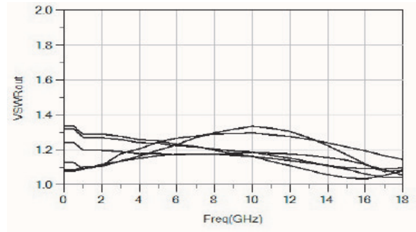
输出驻波
