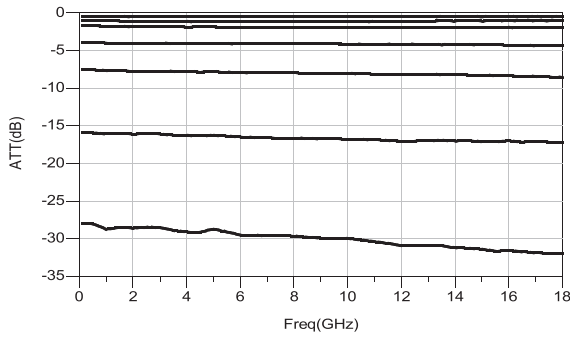
衰减量
