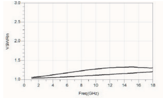
输入驻波
