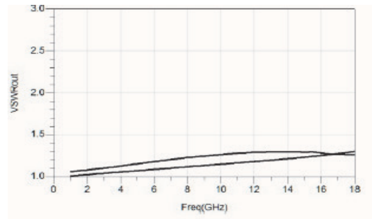
输出驻波
