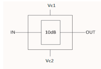
YAT15-01181C1框图
