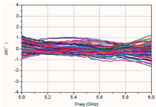
移相精度
