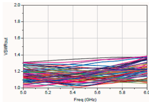
输出驻波
