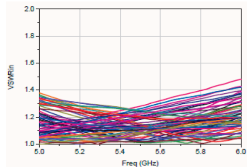
输入驻波
