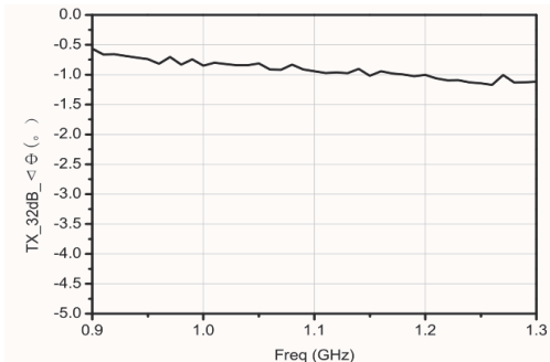
发射 32dB 衰减附加相移
