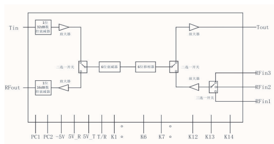
YCC11-01026C1 结构框图
