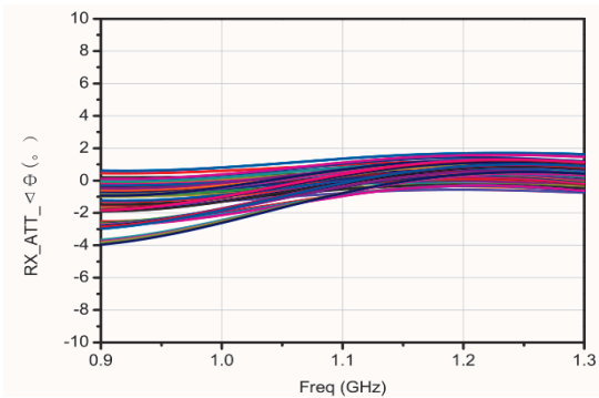
接收衰减态相位波动
