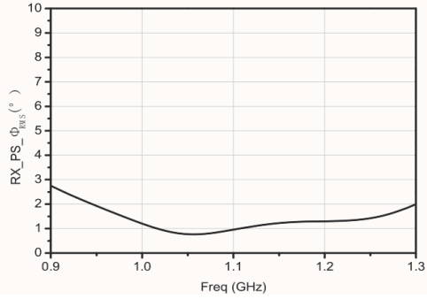
接收移相精度均方根
