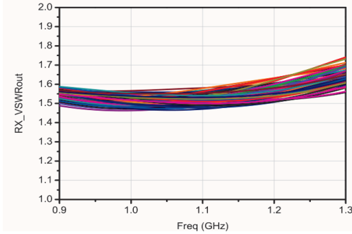
接收输出驻波
