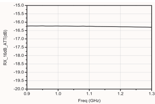
接收 16dB 衰减值
