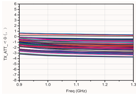
发射衰减态相位波动
