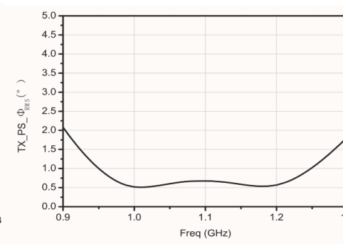
发射移相精度均方根
