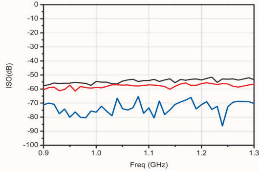
接收 RFin1~RFin3 隔离度
