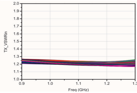
发射输入驻波
