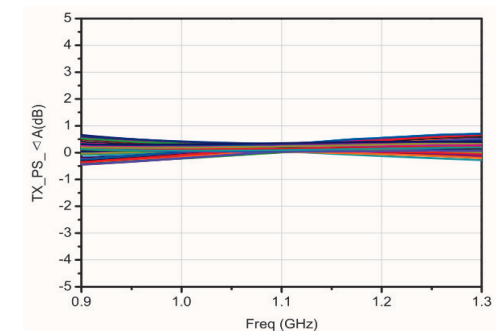
发射移相态幅度变化
