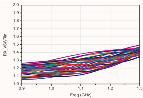
接收输入驻波
