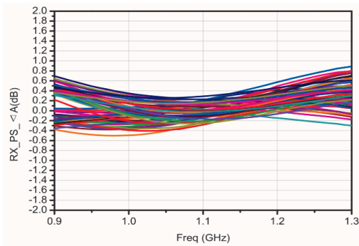
接收移相态幅度变化
