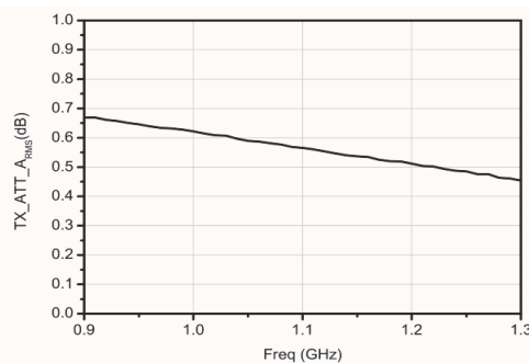
发射衰减精度均方根
