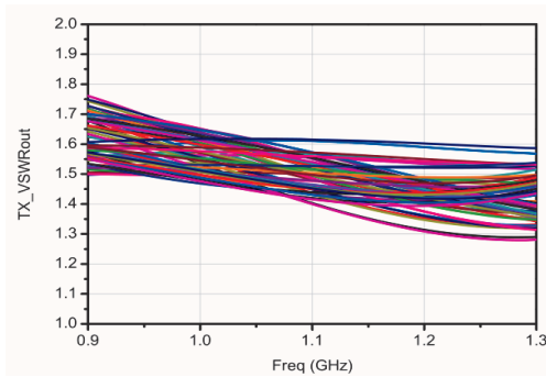
发射输出驻波
