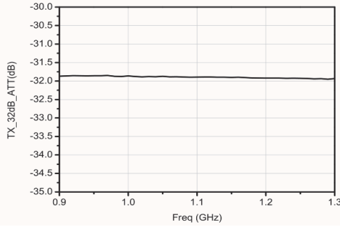
发射 32dB 衰减值
