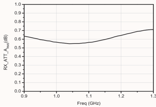
接收衰减精度均方根
