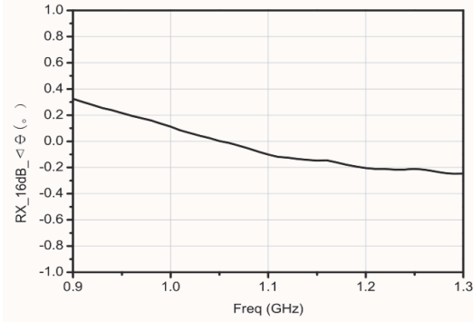
接收 16dB 衰减附加相移
