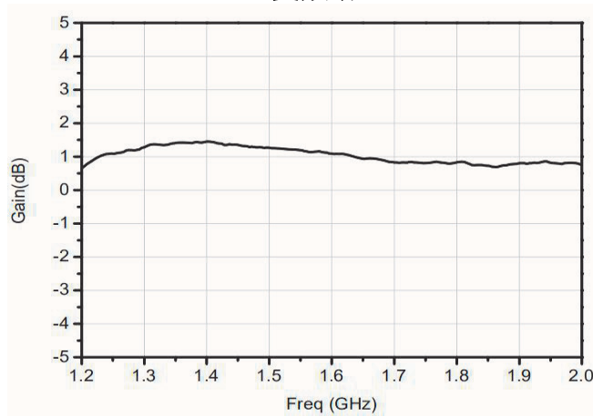
变频增益
