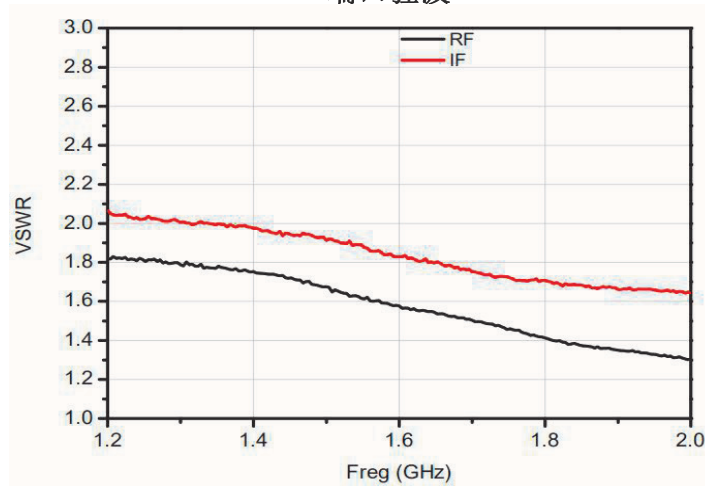
端口驻波
