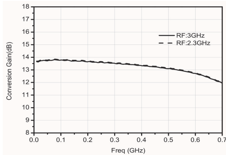
变频增益(LO=0dBm)
