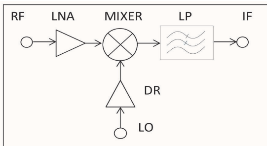
功能框图
