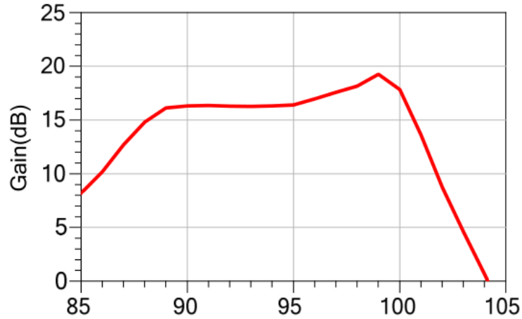
小信号增益vs.频率
