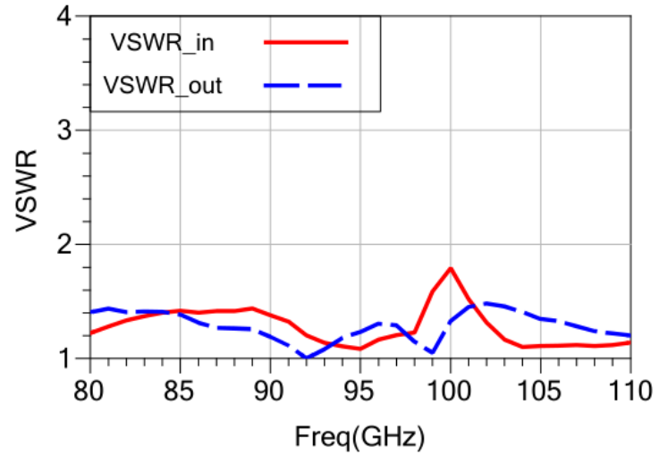
输入/输出驻波vs.频率
