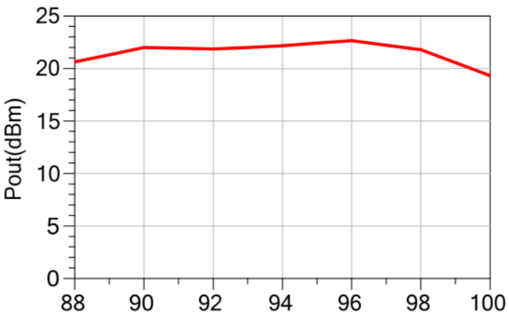
饱和输出功率 vs.频率@Pin=6dBm
