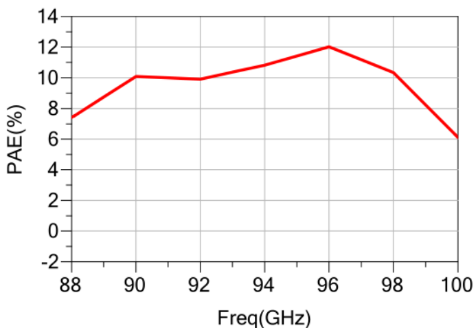
功率附加效率 vs.频率@Pin=6dBm
