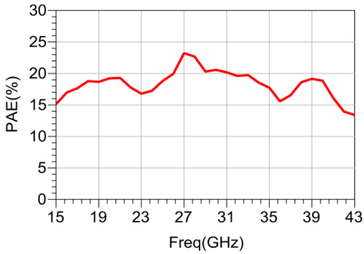
功率附加效率 vs. 频率 @ Pin=12dBm
