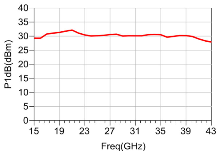
P1dB vs.频率
