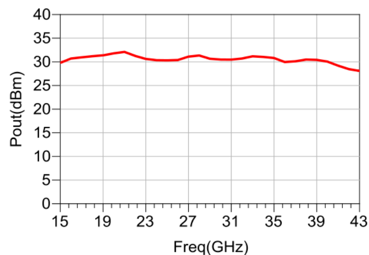
饱和输出功率vs.频率 @Pin=12dBm
