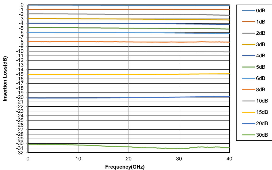
插入损耗 vs. 工作频率
