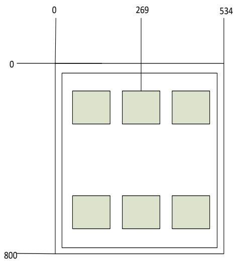
芯片尺寸图 (μm)
