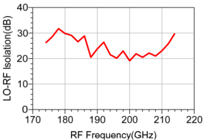
本振-射频隔离度 vs. 射频频率
