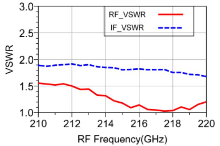
射频/中频驻波 vs. 射频频率
