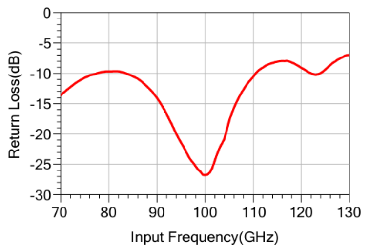
输入回波损耗 vs.频率
