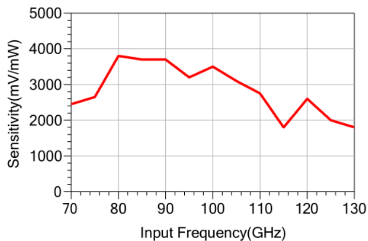
检波灵敏度 vs.频率@Pin=-25dBm
