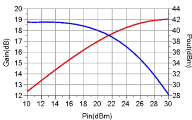
输出功率、功率增益、电流 vs. 输入功率 (33GHz)
