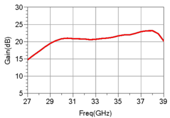
小信号增益 vs. 频率
