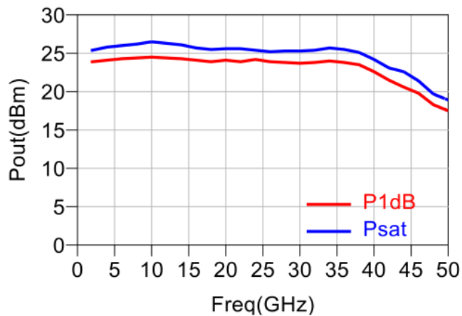
输出功率vs.频率@T A =25°C
