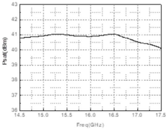
和输出功率 vs. 频率 ( P_{in} = 19\text{dBm} )
