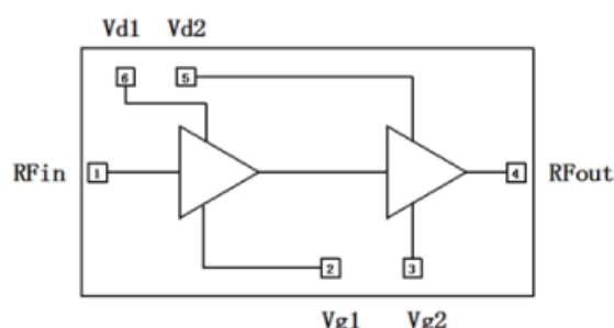
YGPA20-0218C1 功能框图
