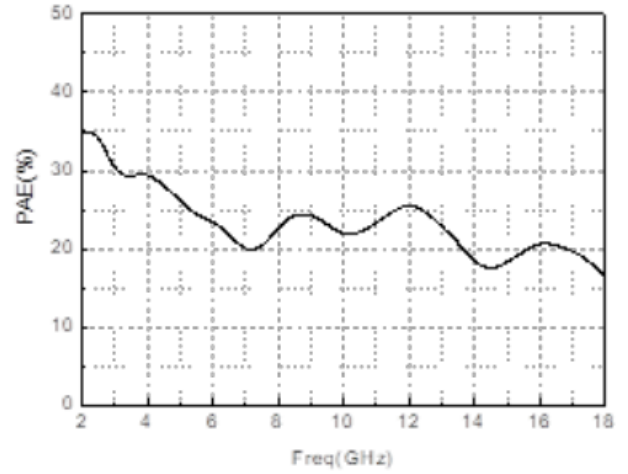
功率附加效率 vs. 频率 ( P_{in} = 28\text{dBm} )
