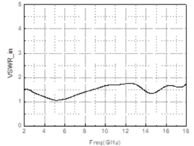
输入驻波 vs. 频率
