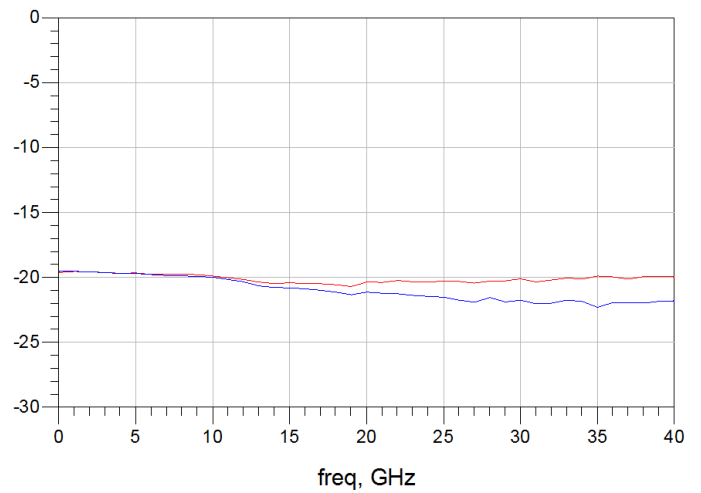
回波损耗
