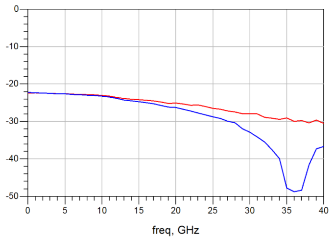
回波损耗
