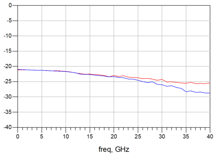
回波损耗
