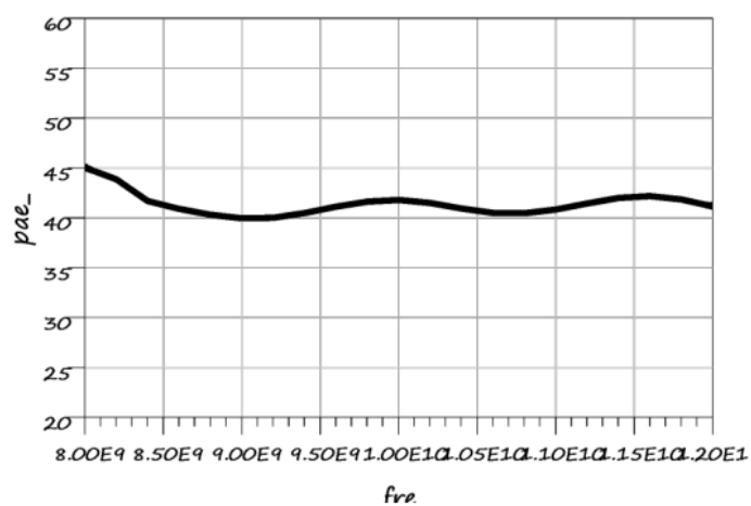
附加效率 vs. 频率 ( P_{in} = 19\text{dBm} )
