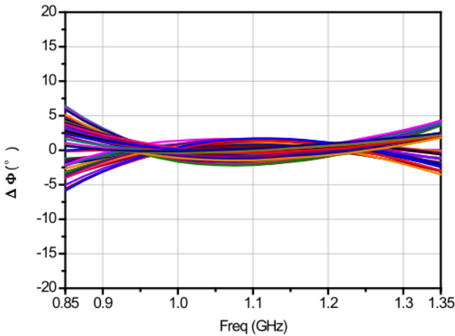
移相精度
