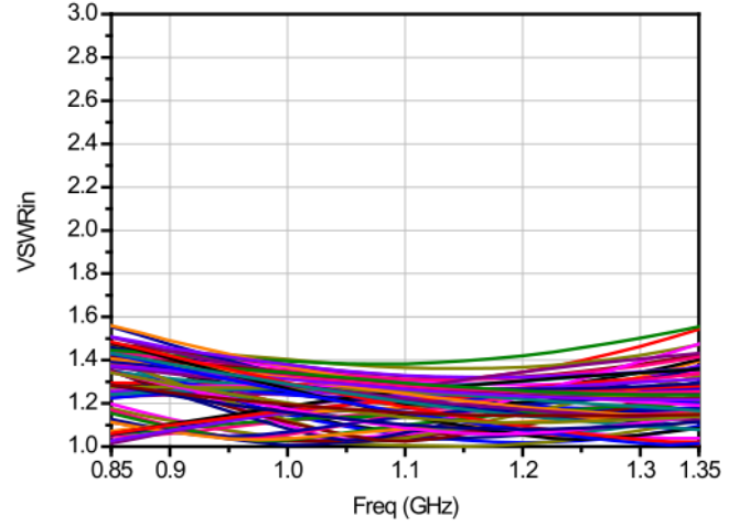
输入驻波
