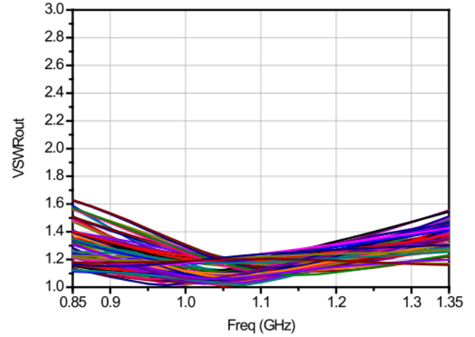
输出驻波
