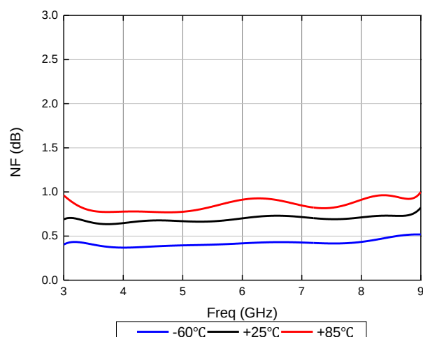
噪声系数
