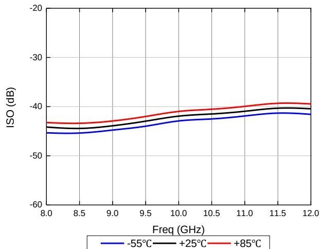
RFC-RF2隔离度
