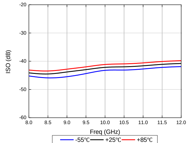
RFC-RF1隔离度
