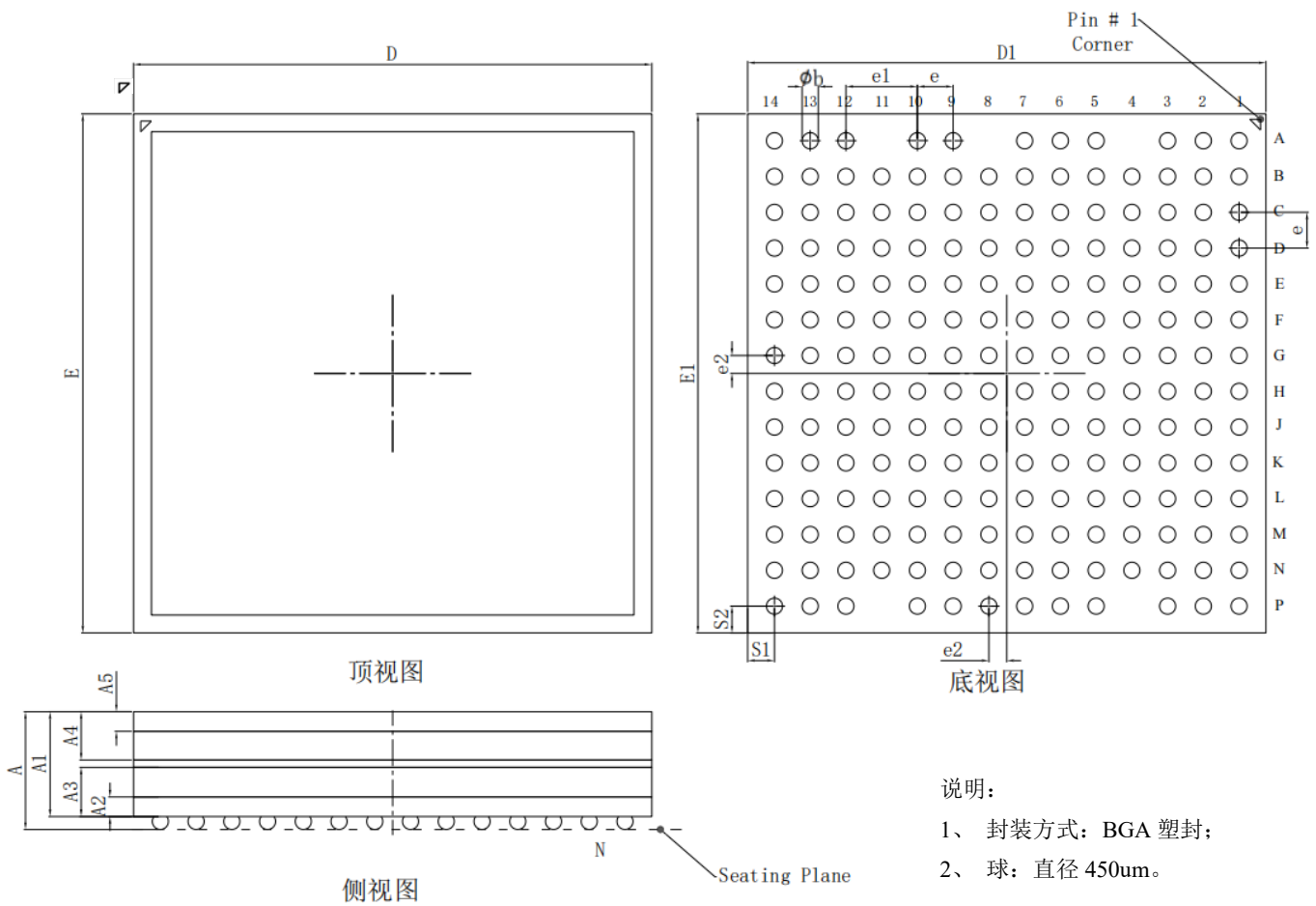
外形结构图 (单位: mm)
