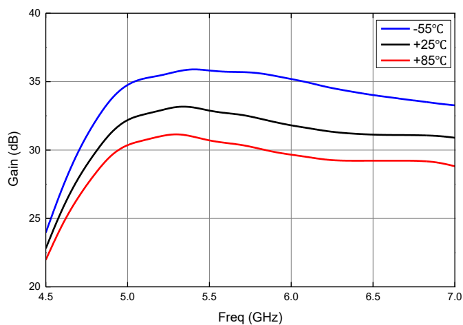
小信号增益 (Pulse)
