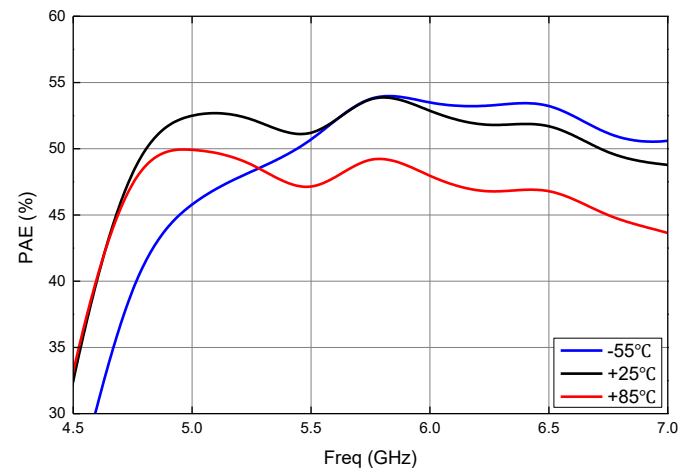
功率附加效率 (CW)
