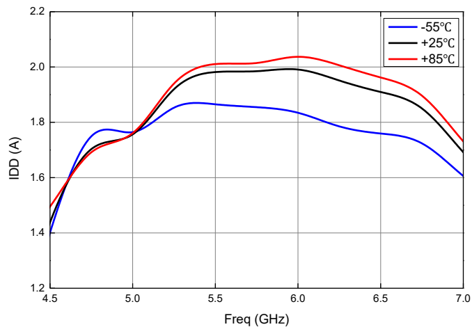
动态电流 (Pulse)
