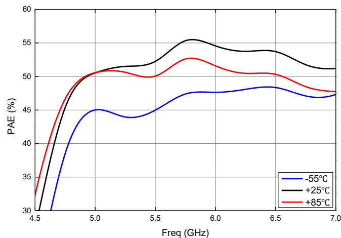
功率附加效率 (Pulse)
