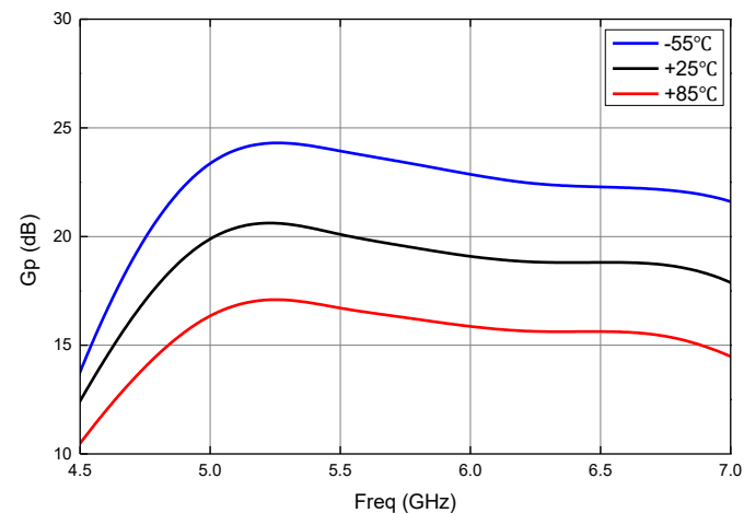
功率增益 (CW)
