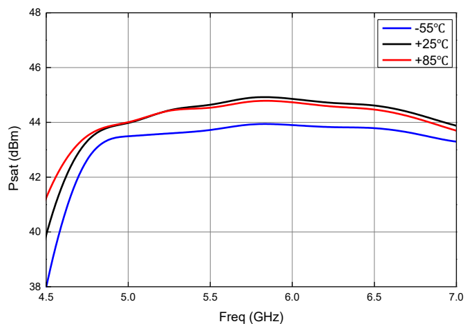
饱和输出功率 (Pulse)
