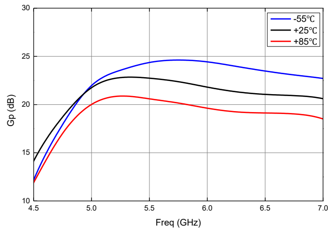
功率增益 (Pulse)
