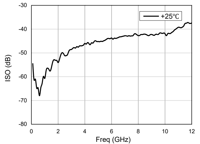
反向隔离度
