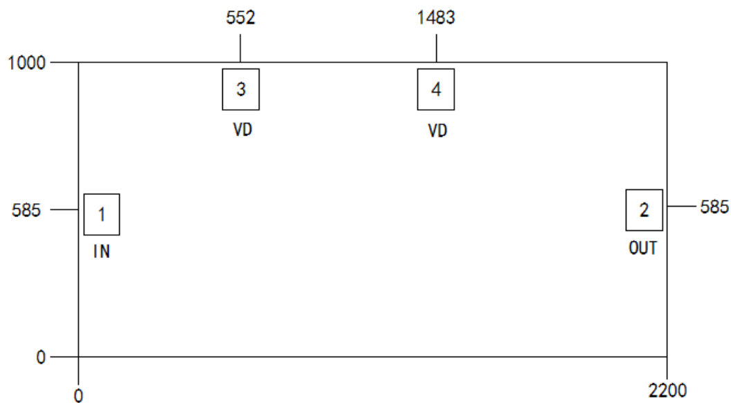
芯片端口图 (单位: \mu\text{m} )
