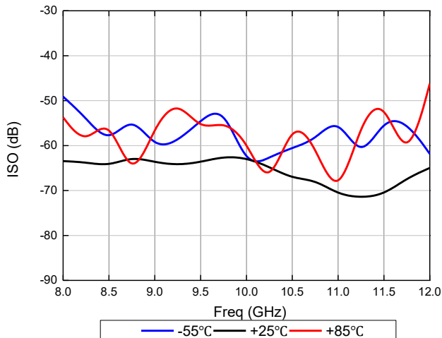
隔离度 (Pulse)
