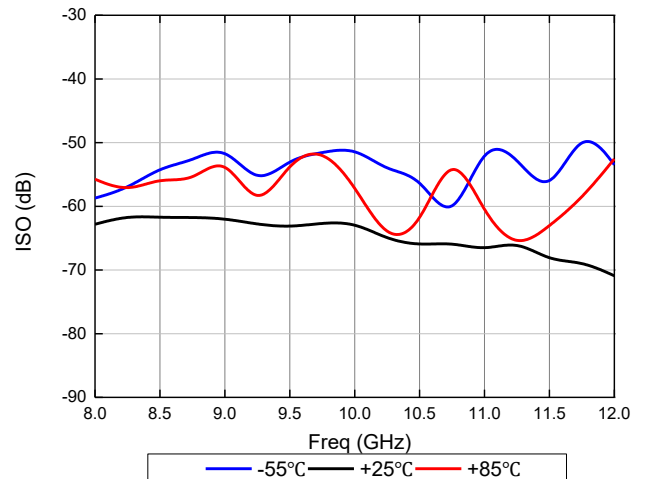
隔离度 (CW)
