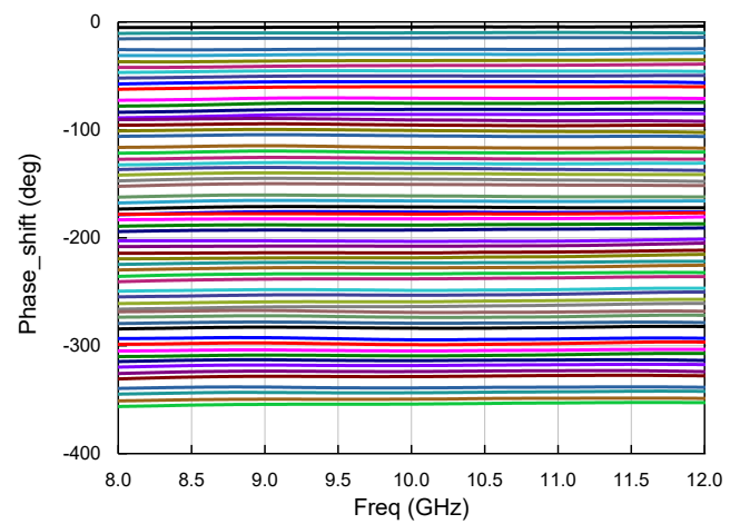
全态移相量
