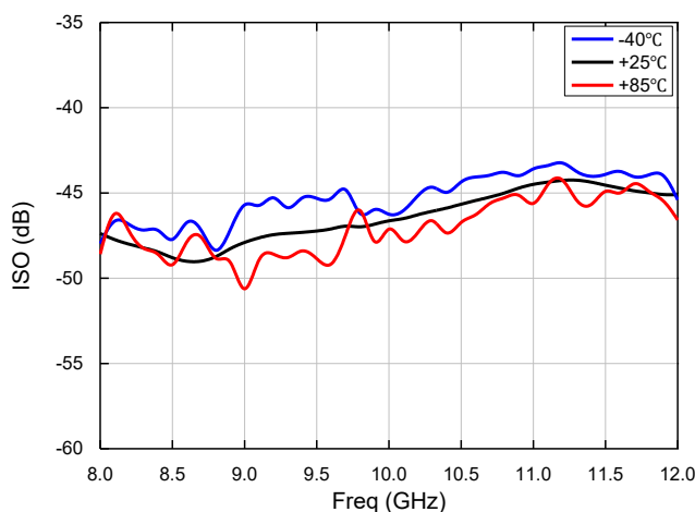
RF1-RF2隔离度
