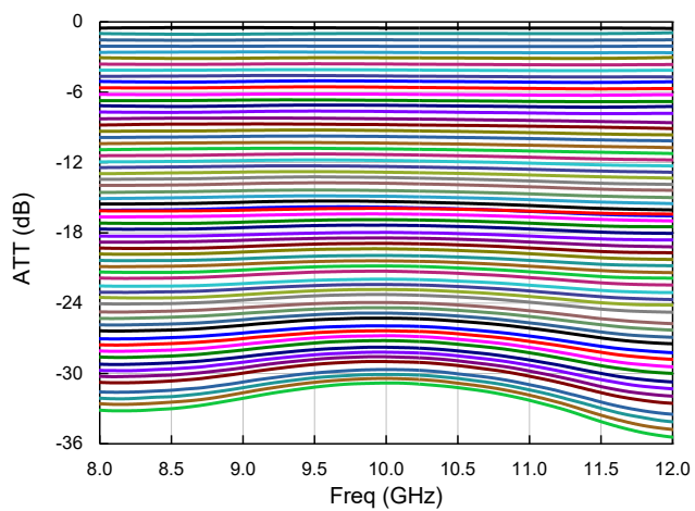
全态衰减量
