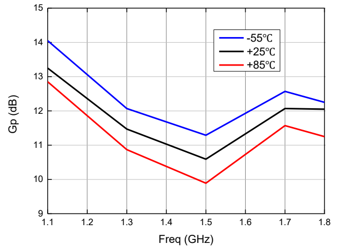
功率增益
