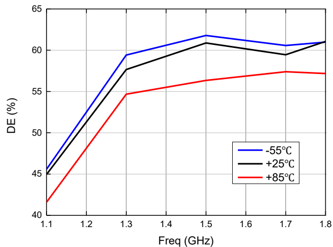
漏极效率
