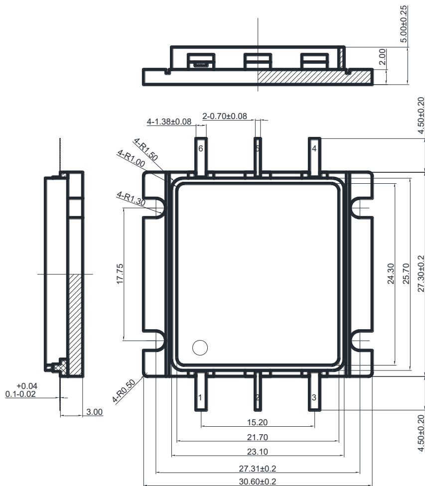
外形尺寸图 (单位: mm)
