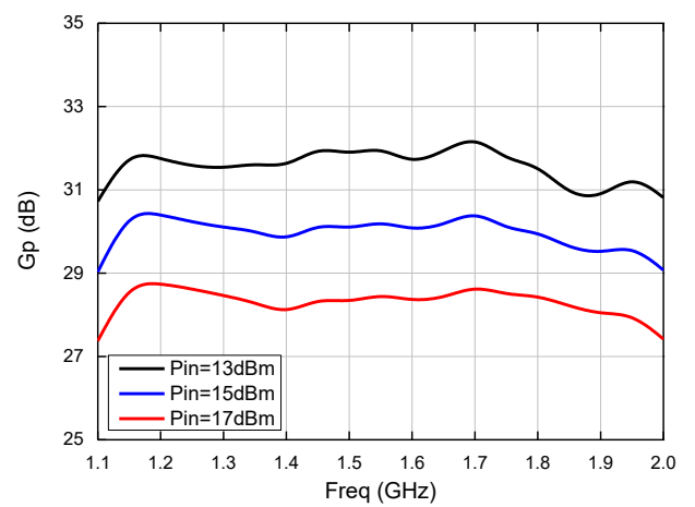
功率增益
