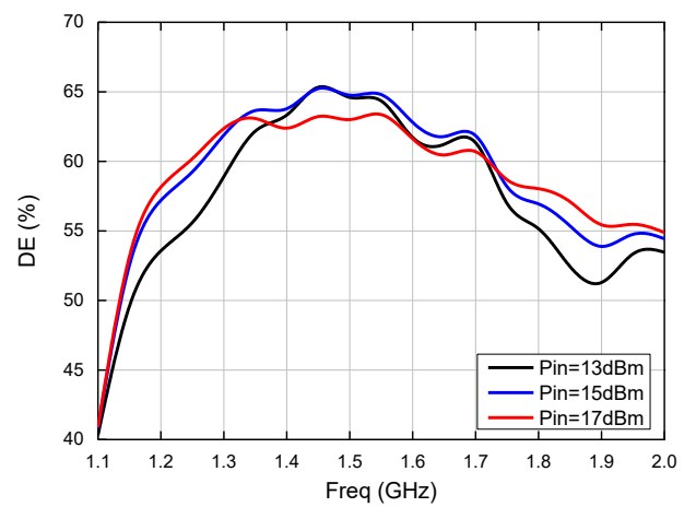
漏极效率
