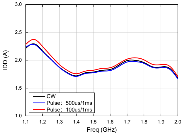
动态电流
