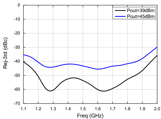
三次谐波抑制
