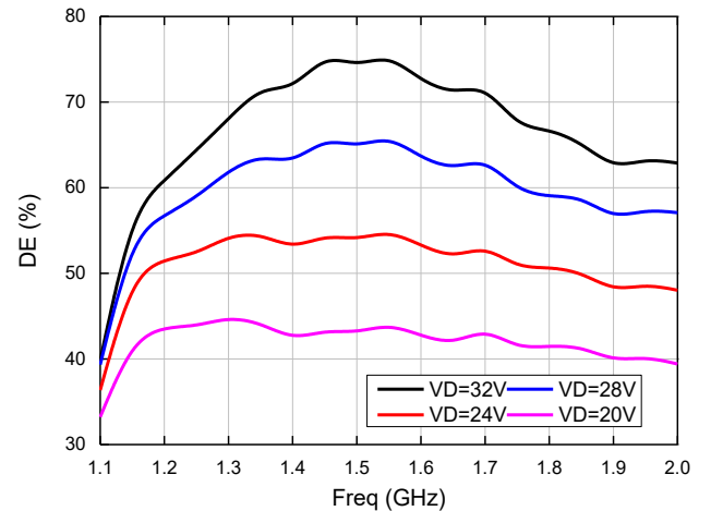
漏极效率
