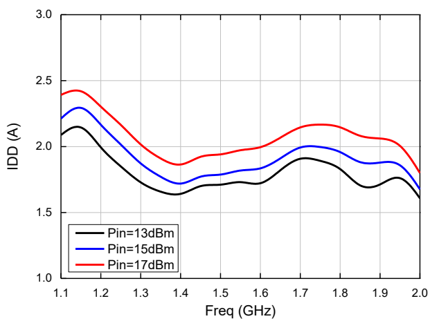
动态电流
