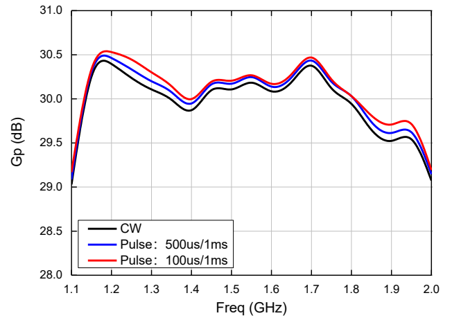
功率增益
