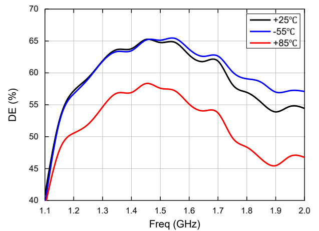
漏极效率
