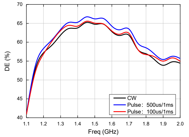
漏极效率
