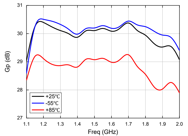
功率增益
