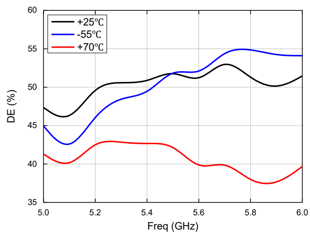
漏极效率
